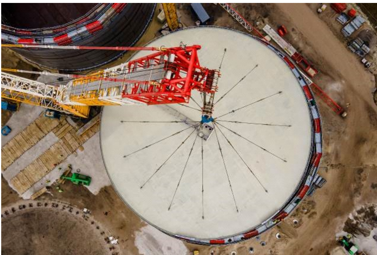
Budowa zbiorników PERN w Nowej Wsi Wielkiej
