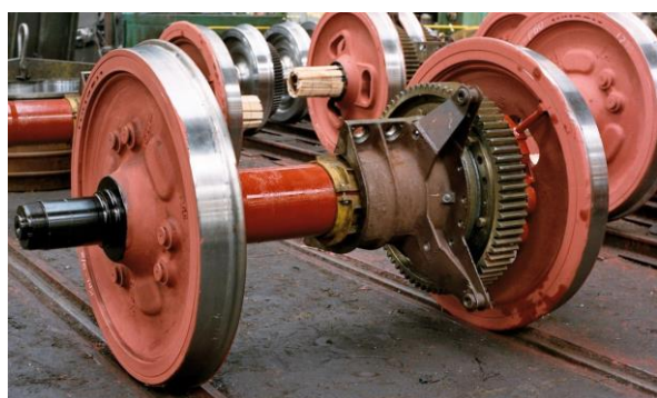
Zestaw kołowy do lokomotyw elektrycznych i spalinowych
